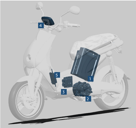
1 Batería. 2 Motor. 3 Controlador. 4 Cuadro de intrumentos. 5 Transformador 12V.
